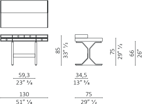
Nòs con cassetti / with drawers
