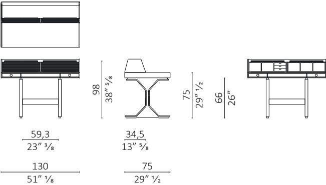
Nòs con serrande / with roll top
